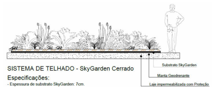
DETALHE 01 1:100
