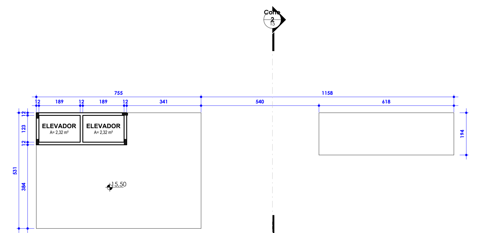
2 PLANTA 5º PAVIMENTO 1 : 100
