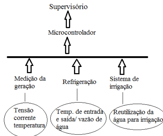
Figura 6. Informações enviadas e ações de cada atuador
