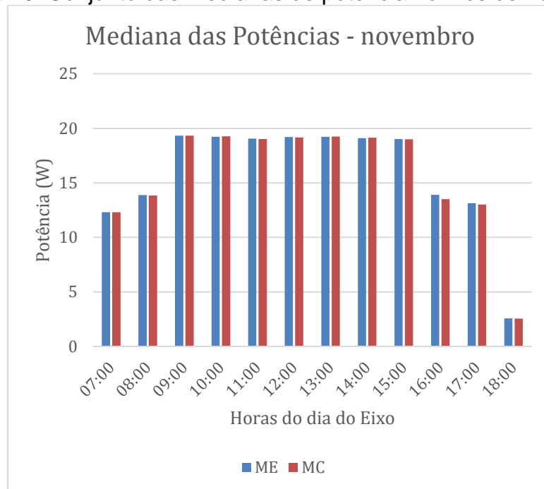
Figura 16. Conjunto das medianas de potência no mês de novembro
