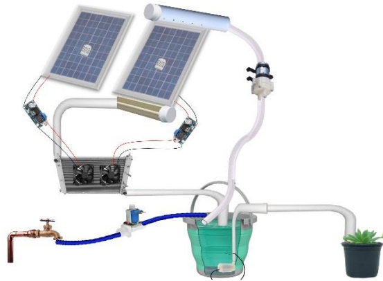
Figura 1. Configuração experimental do sistema
