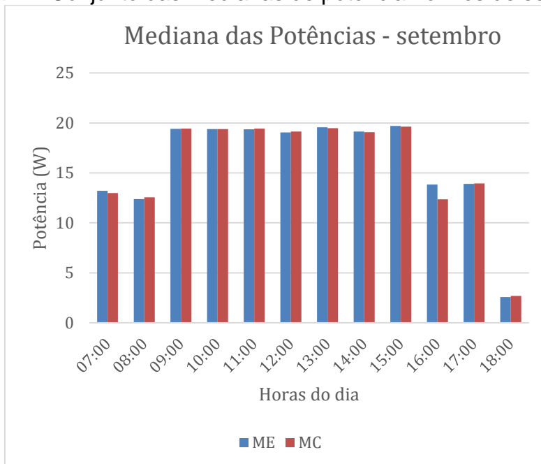
Figura 14. Conjunto das medianas de potência no mês de setembro
