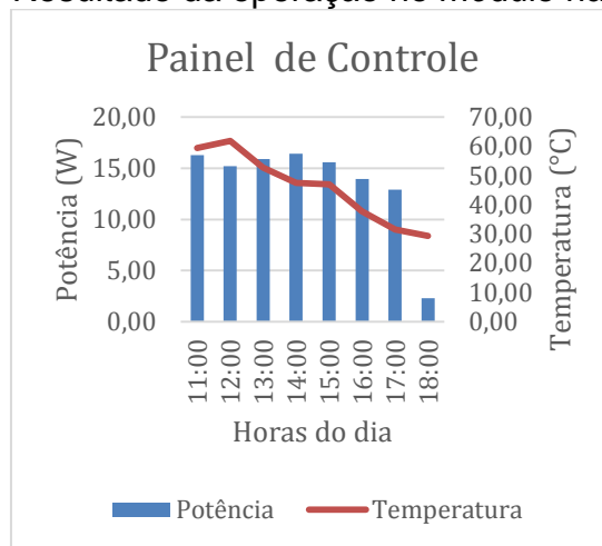
Figura 11. Resultado da operação no módulo não arrefecido
