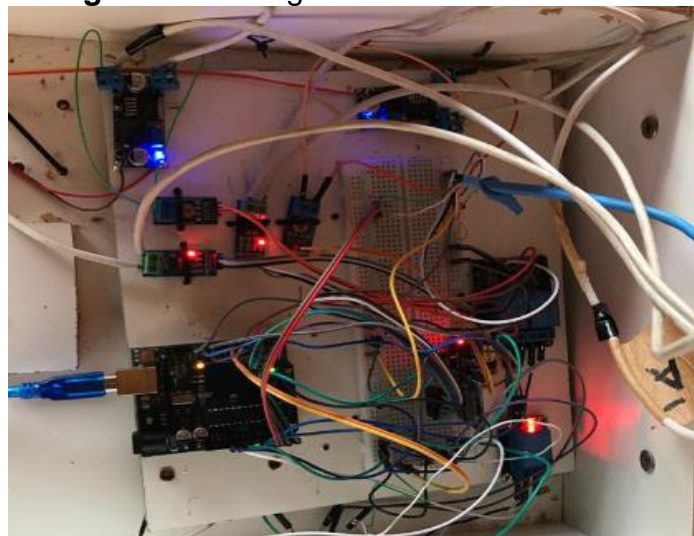
Figura 7. Montagem eletrônica do sistema
