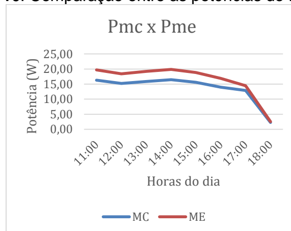
Figura 10. Comparação entre as potências do MC e ME
