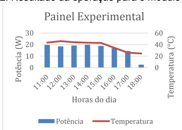
Figura 12. Resultado da operação para o módulo arrefecido
