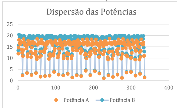
Figura 17. Gráfico de dispersão das potências dos módulos em função da hora (mês de novembro).
