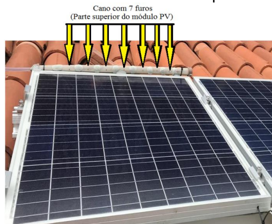
Figura 2. Cano com sete furos sob o painel refrigerado
