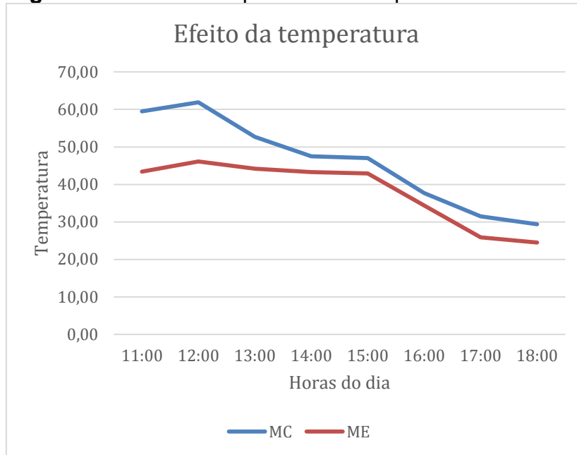
Figura 9. Efeito da temperatura sob o plano dos módulos
